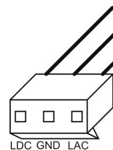
Rys.2 Schemat podłączenia modułu do zasilacza PSB.
